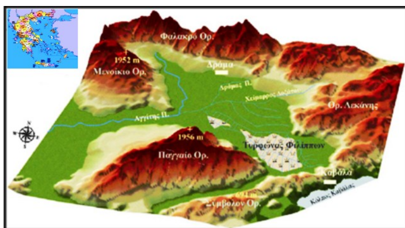
Σχηματική τρισδιάστατη απεικόνιση της Λεκάνης της Δράμας
